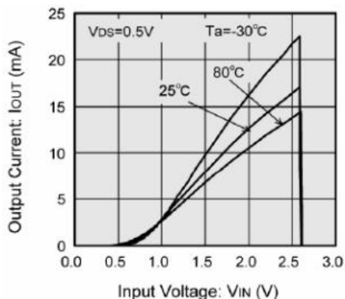
5. N 管漏开路输出电流 与输入电压
