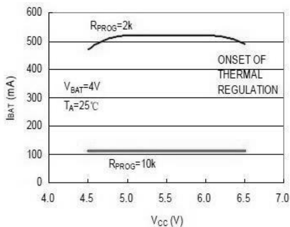
充电电流 VS 电源电压
