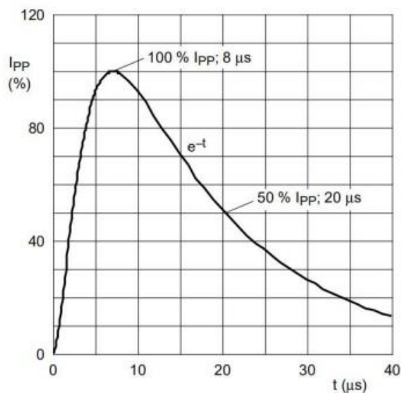
IEC 61000-4-5 Waveform( 8/20 \mu\text{s} pulse)
